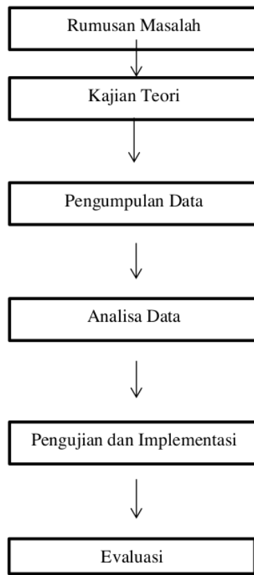
Gambar 1. Metodologi Penelitian
