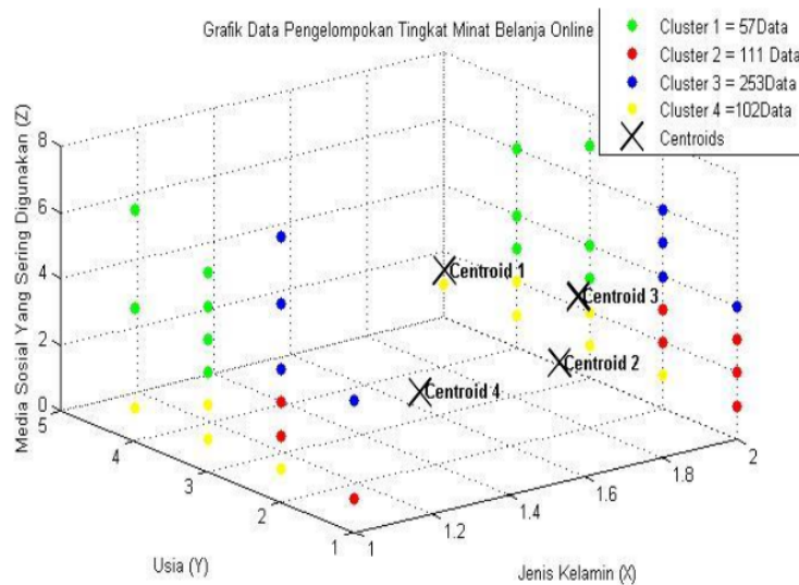
Gambar 4. Grafik 4 Cluster
