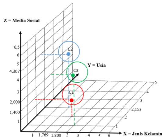
Gambar 2. Grafik Clustering
