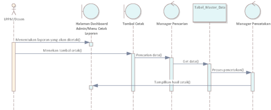
Gambar 14. Sequence Diagram Cetak Laporan
