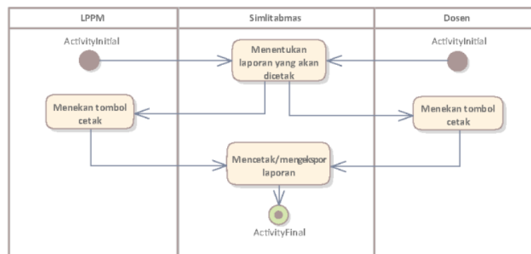
Gambar 8. Activity Diagram Cetak Laporan
