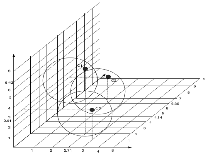
Gambar 2 Grafik Cluster
