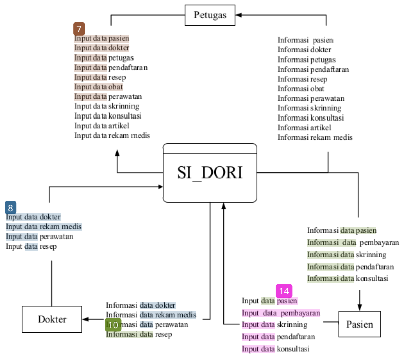
Gambar 1. Diagram Konteks Perancangan Database
