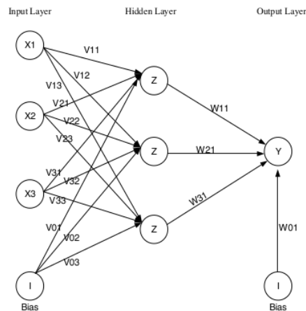
Gambar 1. Arsitektur JST
