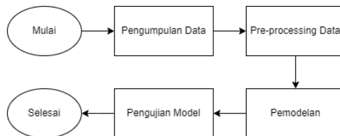
Gambar 2.1. Tahapan Penelitian
