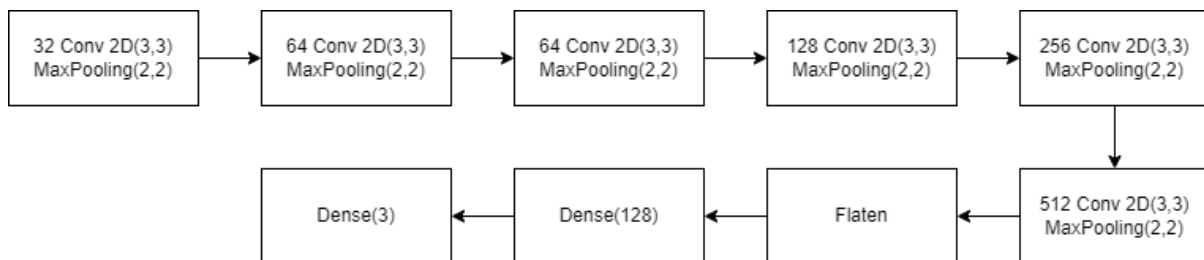
Gambar 2.4. Arsitektur CNN
