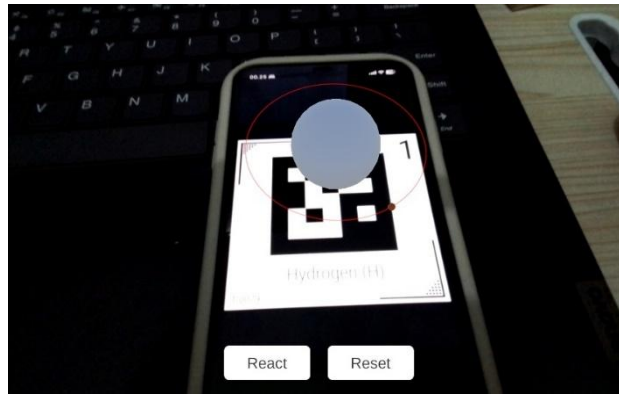
Gambar 4.9 Halaman Utama
