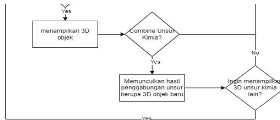
Gambar 4.1 Flowchart Aplikasi
