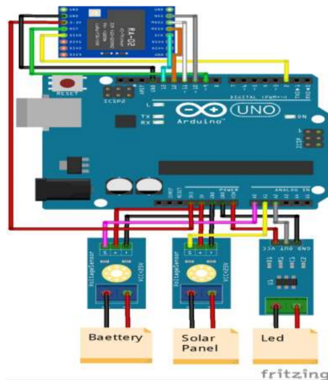
Gambar 5. Skematik
