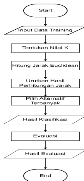
Gambar 2 Skema KNN
