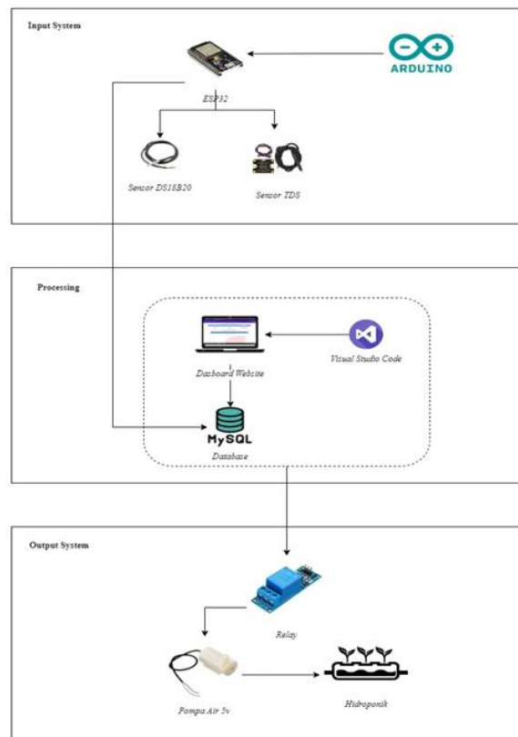
Gambar 1. Desain Sistem
