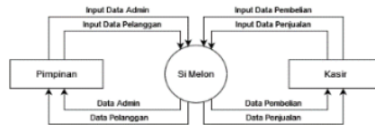
Gambar 15. Diagram Konteks
