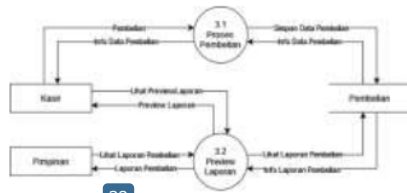
Gambar 19. DFD Level 2 Pembelian
