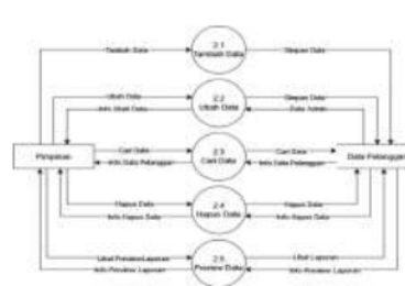
Gambar 17. DFD Lvl 2 Data Admin Gambar 18. DFD Lvl 2 Data Pelanggan
