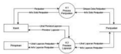
Gambar 20. DFD Level 2 Penjualan
