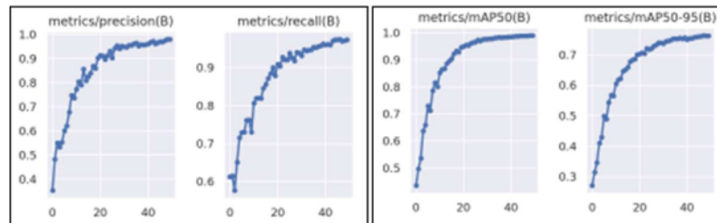
Gambar 4.7. Grafik Performa Precision, Recall , dan mAP
