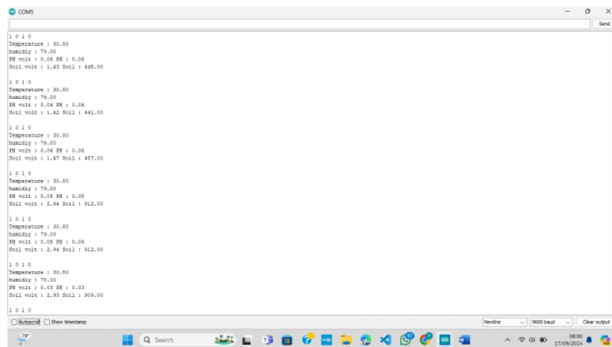
Gambar IV.9 Tampilan pada Serial Monitor
