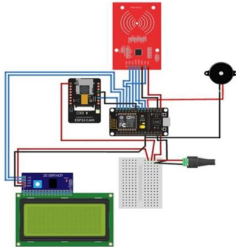
Gambar 7. Skema Rangkaian
