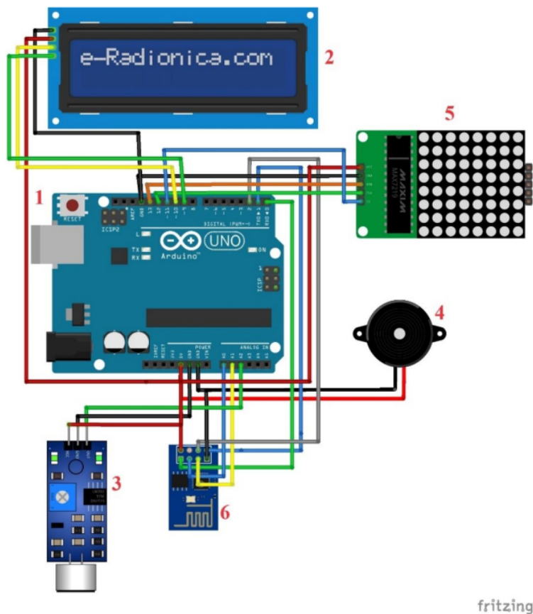
Gambar 8. Skema Rangkaian
