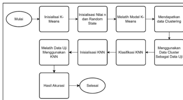
Gambar 4. Perancangan Model K-Means dan KNN
