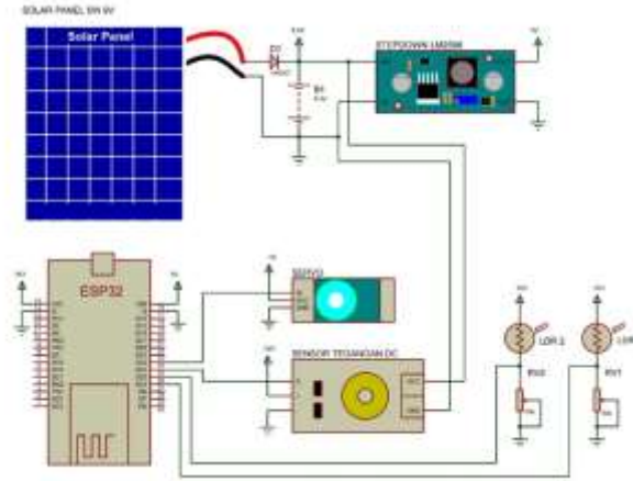
Gambar 8. Skema Rangkaianasaasa
