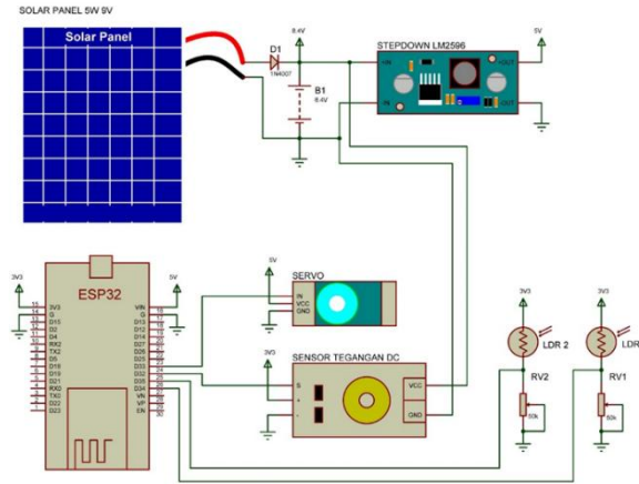
Gambar 8. Skema Rangkaianasaasa
