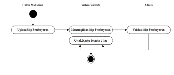
Gambar 6. Activity Diagram Mencetak Kartu Peserta Ujian
