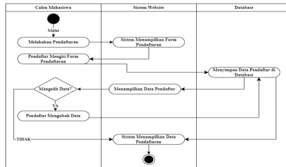
Gambar 5. Activity Diagram Mengisi Data Diri
