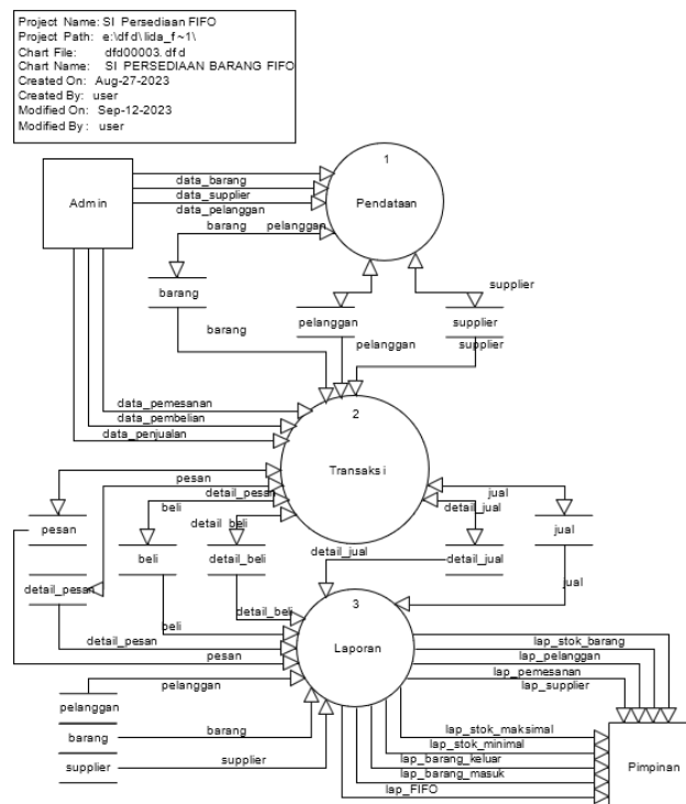
Gambar 3.4 DFD Level 0
