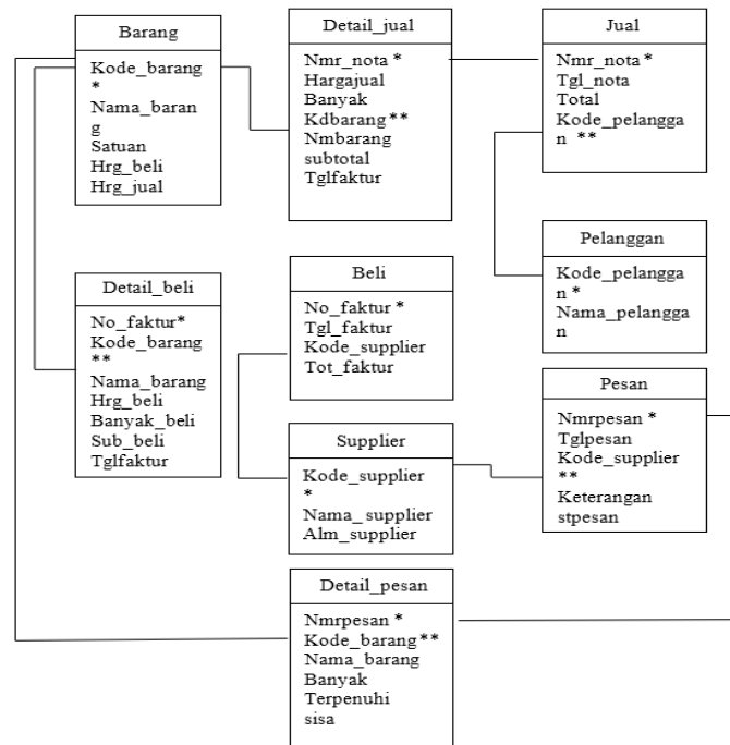
Gambar 3.5 normalisasi ke 3
