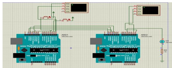
Gambar 2. Analisis komunikasi SPI
