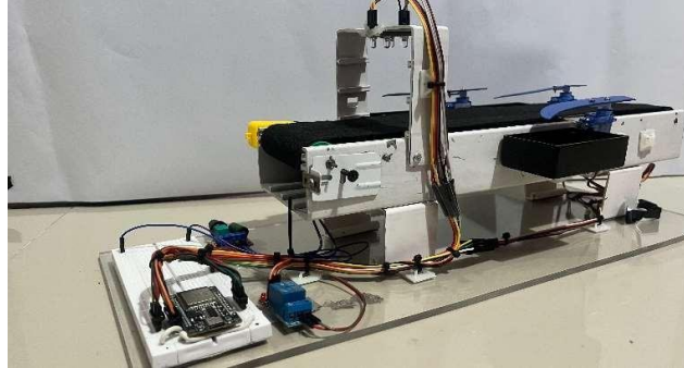
Gambar 5. Mini Conveyor
