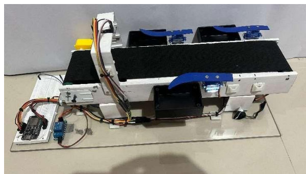
Gambar 7. Pengujian Mini Conveyor
