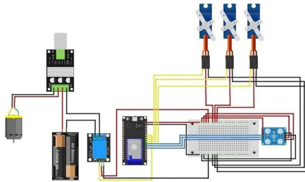
Gambar 2. Diagram Rangkaian
